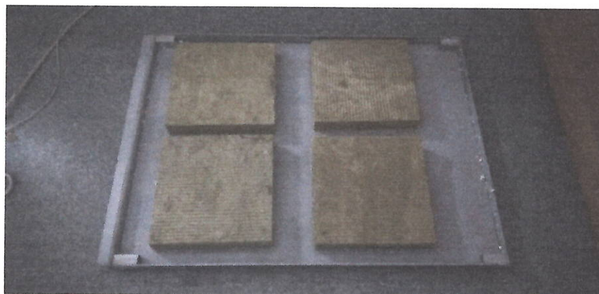
Рисунок 8 – Зволоження дослідних зразків теплоізоляційного матеріалу марки «ТЕХНОВЕНТ Н»
