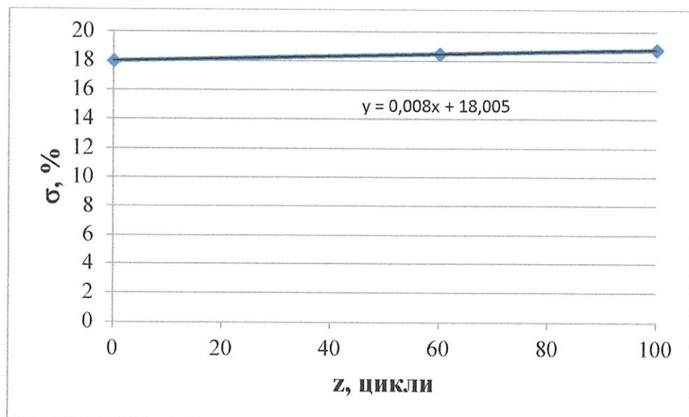
Рисунок 6 – Залежність міцності на стиск при 10% деформації від циклічних впливів зразків теплоізоляційного матеріалу марки «ТЕХНОВЕНТ Н»
